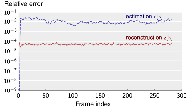
(d) Hall (noisy case): Relative errors of estimation and reconstruction.
